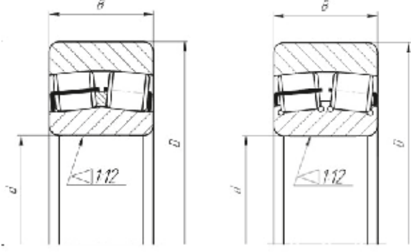
СФЕРИЧЕСКИЕ ДВУХРЯДНЫЕ РОЛИКОВЫЕ ПОДШИПНИКИ НА ВНУТРЕННЕМ КОЛЬЦЕ С КОНИЧЕСКИМ ОТВЕРСТИЕМ, КОНУСНОСТЬЮ 1:12 Внутренняя конструкция: с суффиксом К
