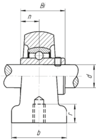
КОРПУСНЫЕ ПОДШИПНИКОВЫЕ УЗЛЫ СЕРИИ USPA200
