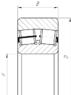
СФЕРИЧЕСКИЕ ДВУХРЯДНЫЕ РОЛИКОВЫЕ ПОДШИПНИКИ С БОРТИКАМИ НА ВНУТРЕННЕМ КОЛЬЦЕ Внутренняя конструкция: с суффиксом CA
