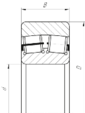
СФЕРИЧЕСКИЕ ДВУХРЯДНЫЕ РОЛИКОВЫЕ ПОДШИПНИКИ С БОРТИКАМИ НА ВНУТРЕННЕМ КОЛЬЦЕ Внутренняя конструкция: с суффиксом СА
