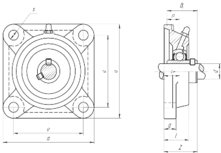
КОРПУСНЫЕ ПОДШИПНИКОВЫЕ УЗЛЫ СЕРИИ UCF200 И UCF300
