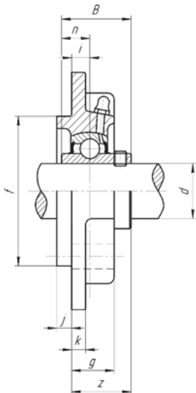
КОРПУСНЫЕ ПОДШИПНИКОВЫЕ УЗЛЫ СЕРИИ УСРА200
